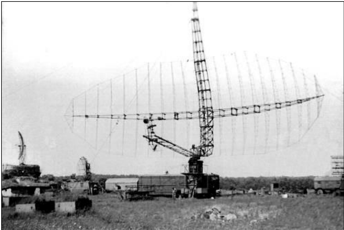
Pildil vasakult: kõrgusemõõtja ПРБ-16, lühimaaradar HP3 73E6 ja kaugmaaradarijaam П-14Ф Autor А. Леонтьев, Autoriõigused ja/või allikas http://14dpvo.ucoz.ru/photo/53-0-985
