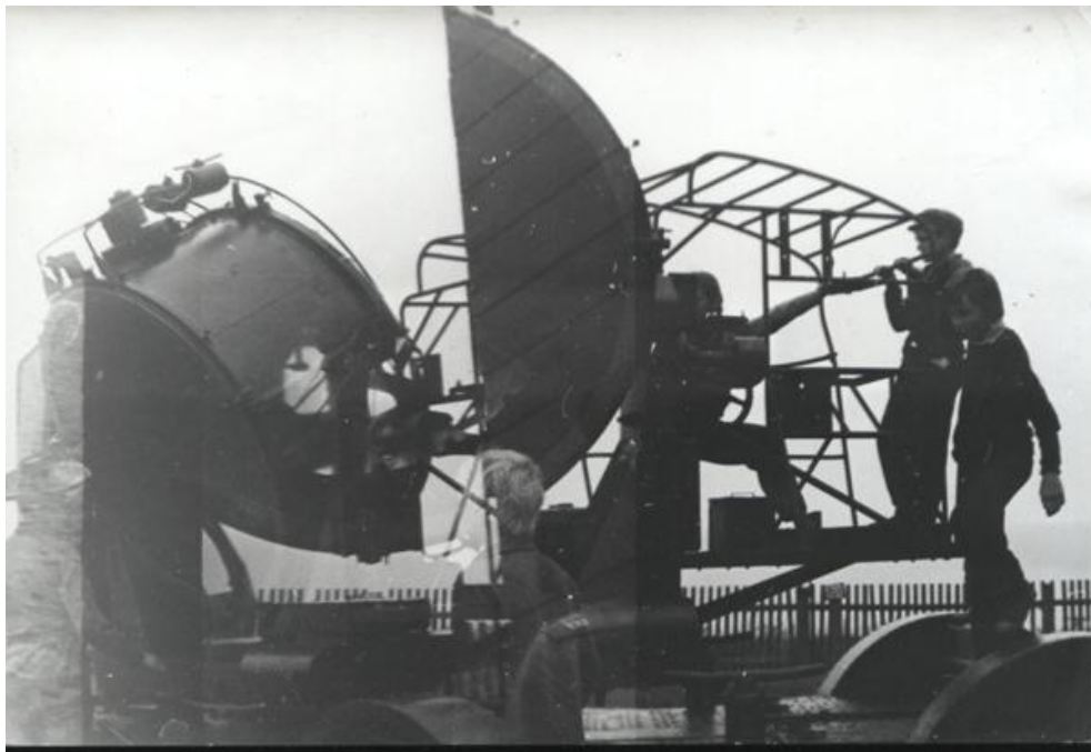
Foto 55. Paljassaare vana tehnilise vaatluse post. Prožektor RP-15-1 positsioonil [22] 1977. a suvel, kordoni šeflusaluse Kopli 8-klassilise kooli piirivalvurite noorte sõpradega. Tollal ümbritses objekti u 1 m kõrgune lippaed. Allikas: http://www.pzokk.narod.ru/index314.html (v. 5.12.2016).
