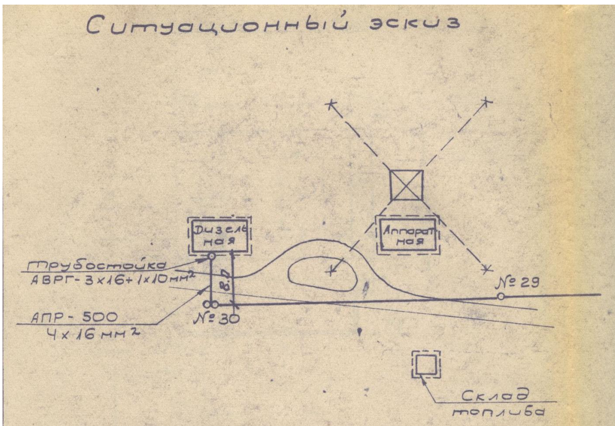
Skeem 8. Paljassaare vana tehnilise vaatluse post. Asendieskiis. Allikas: ÜRPTUI „Energiavõrkude Projekt” Eesti osakond. S/o 2198 Paljassaare poolsaare spetsobjekti elektrivarustuse projekt (autori valduses).
